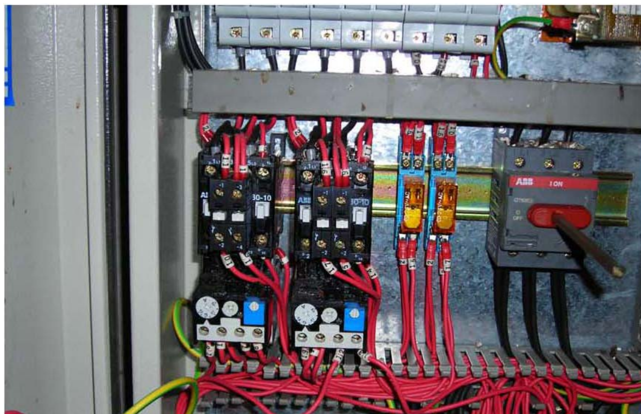
Fotografia 06 – Quadro elettrico
